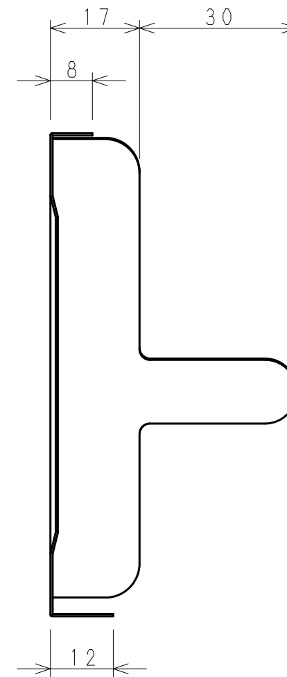
A-A' 断面図
