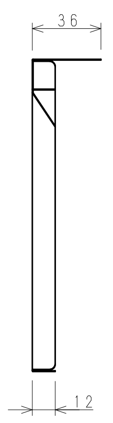
A-A' 断面図
