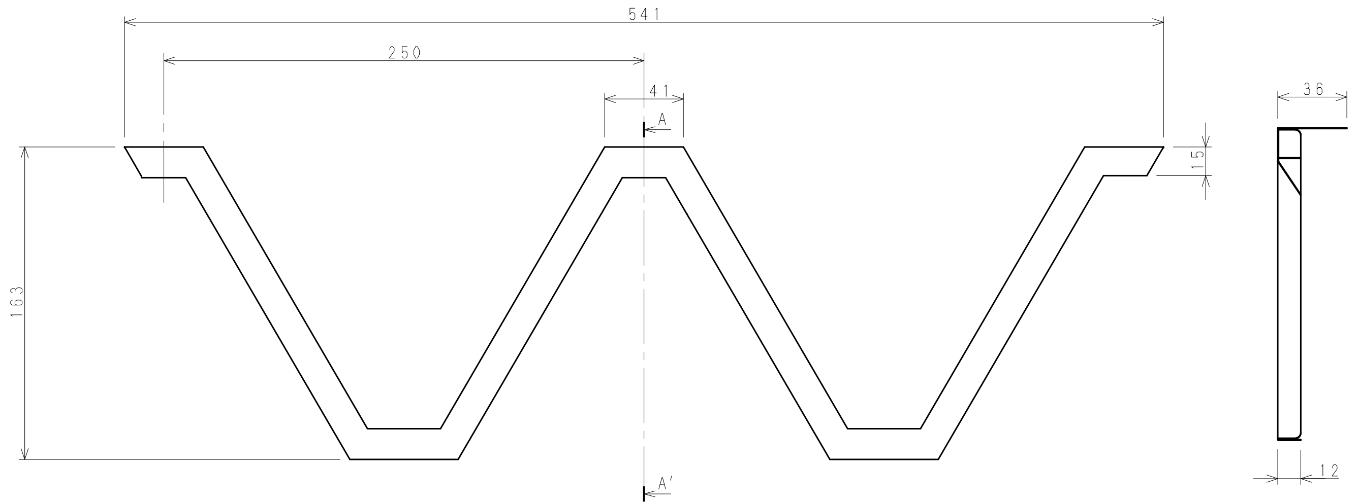
A-A' 断面図
