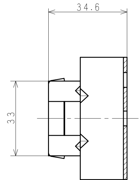
A-A' 断面図
