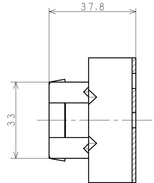
A - A' 断面図
