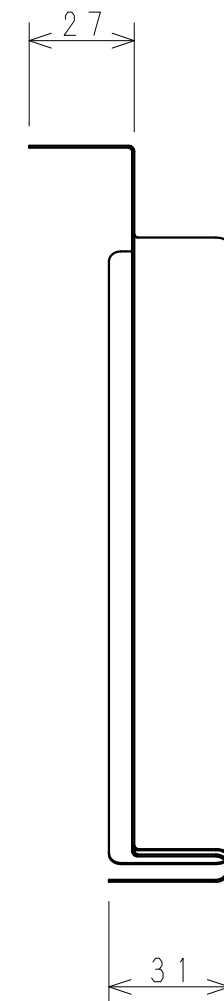
A-A' 断面図
