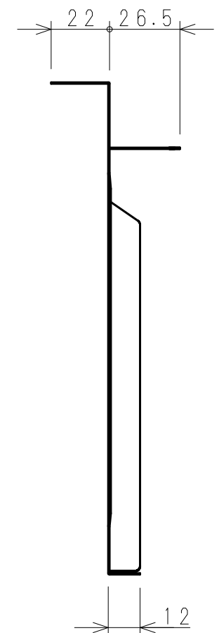
A-A' 断面図
