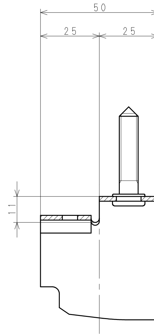
A-A' 断面図
