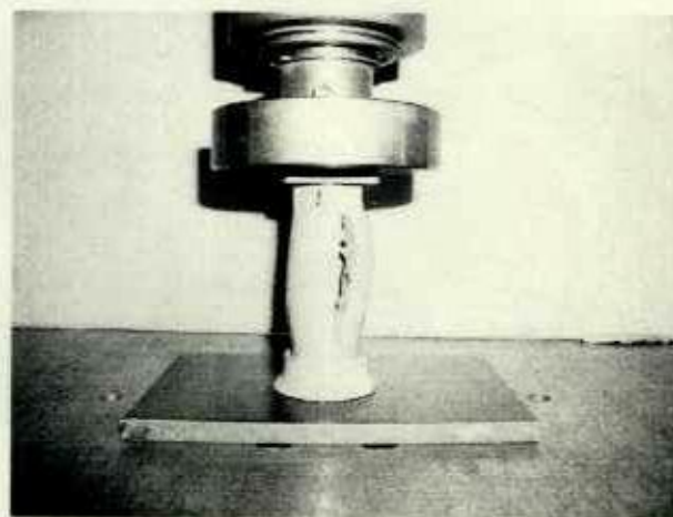
圧縮試験後
