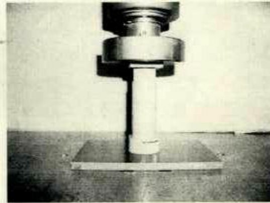
圧縮試験
