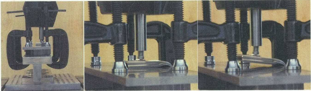
図. 試験の様子 (左 : 全景、中 : 試験前、右 : 試験後)
