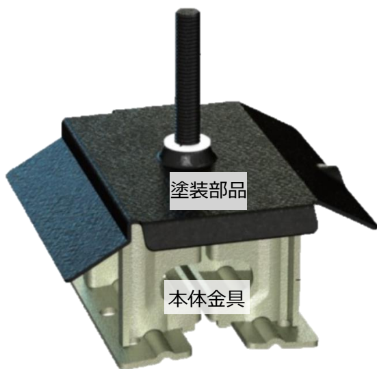
ハゼ式ソーラー金具 高強度タイプ
