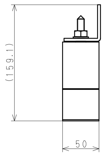
A-A' 断面
