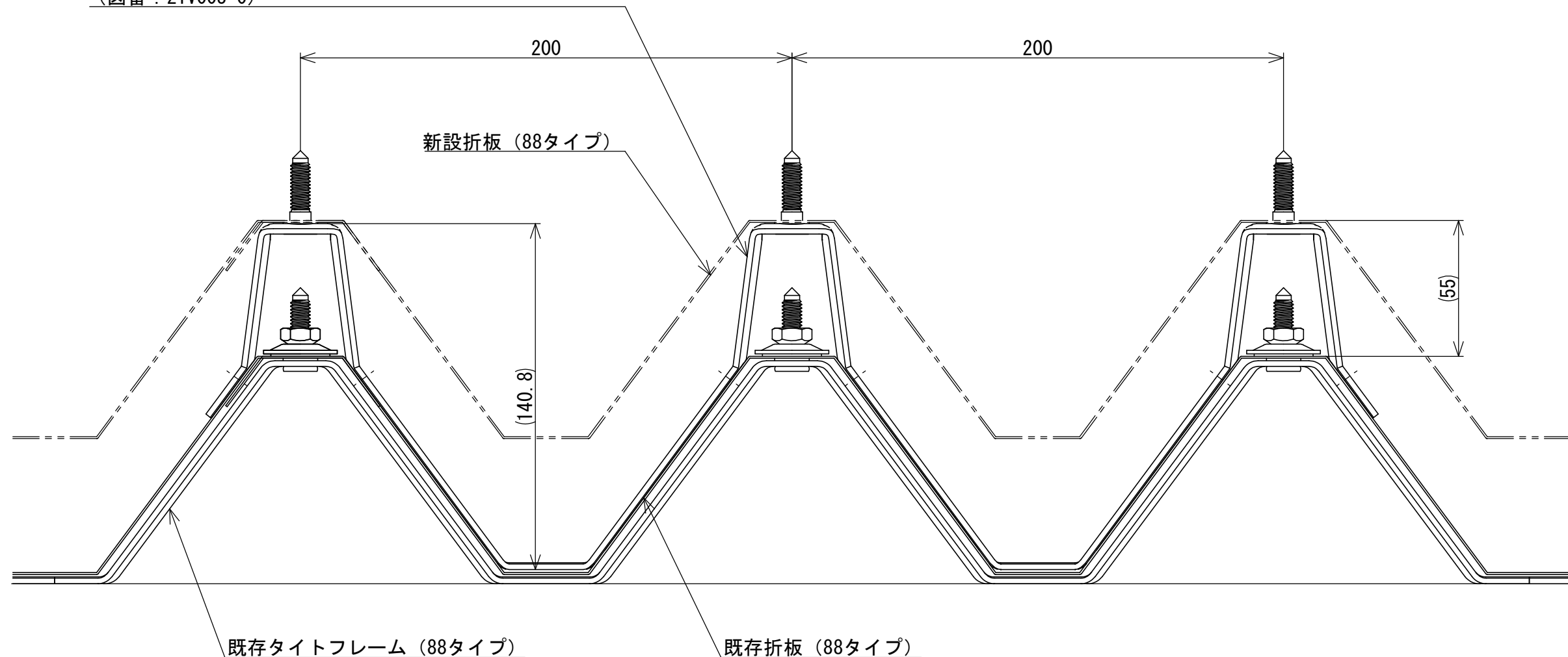
ふき葺Ⅱ型 88ライトタイプ W5/16 RS剣先 ハイセット付 (図番：21V003-0)
