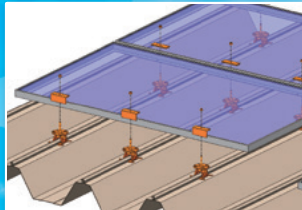
直付工法
