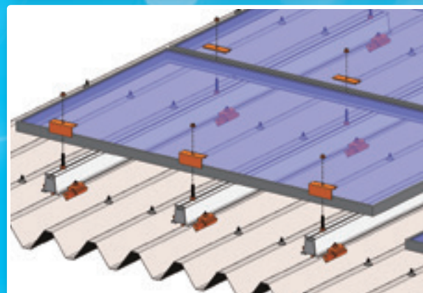
ラック工法
