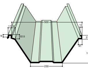
面戸〈H160〉 (標準板厚0.5mm/ 加工可能板厚0.35~0.6mm) ※原板 ガルバリウム鋼板
